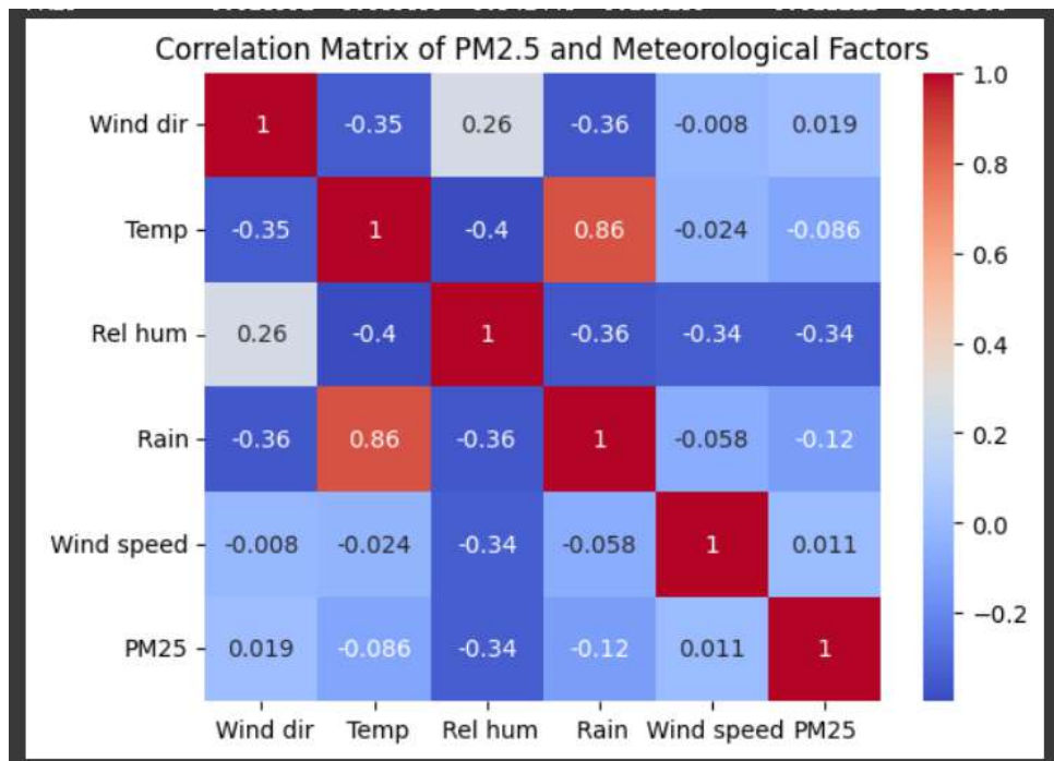
ภาพที่ 9 แสดง Matrix ความสัมพันธ์ตัวแปรกับ PM_{2.5}
