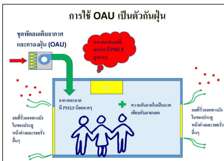
ภาพประกอบ 1 หลักการทำงานของ OAU สร้างห้องสะอาด เครดิตภาพโดย ตุลย์ มณีวัฒนา (2563)
