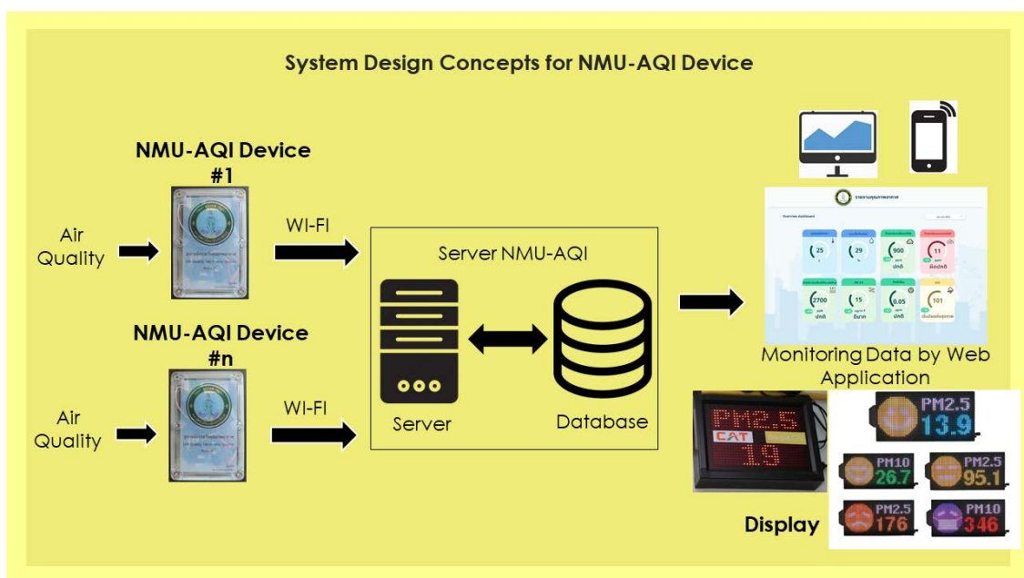
ภาพประกอบ 2 หลักการทำงานของระบบอัตโนมัติตรวจวัดติดตามคุณภาพอากาศ
